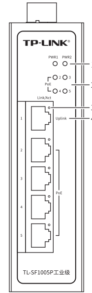
TL-SF1005P工业级 前面板示意图
