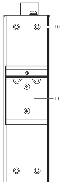
TL-SF1005P工业级 后面板示意图
