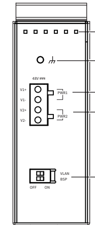
TL-SF1005P工业级 上面板示意图
